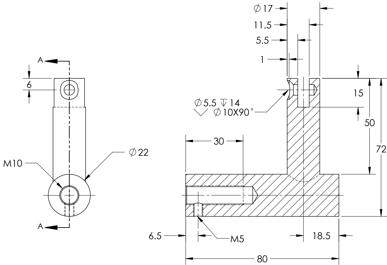
SECTION A-A
